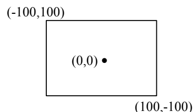
Figura 6.8. Método Scale .
