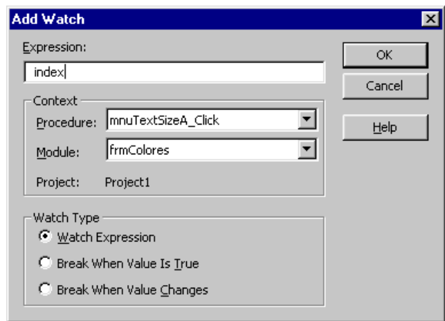
Figura 2.18. Ventana Watches .
