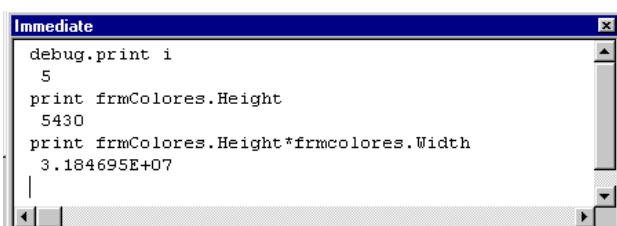
Figura 2.14. Ventana Immediate .
